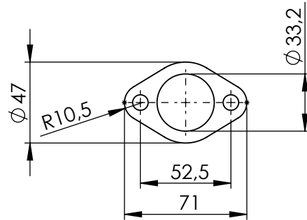
Flange s.s. 43E sp.5mm cod.206308
